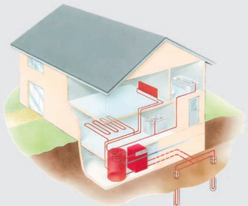
Schematische Darstellung eines Erdsondensystems
